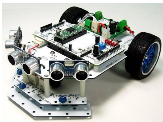
輪型機器人最速挑戰比賽參考作品
