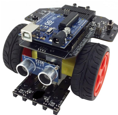
輪型機器人最速挑戰比賽參考作品
